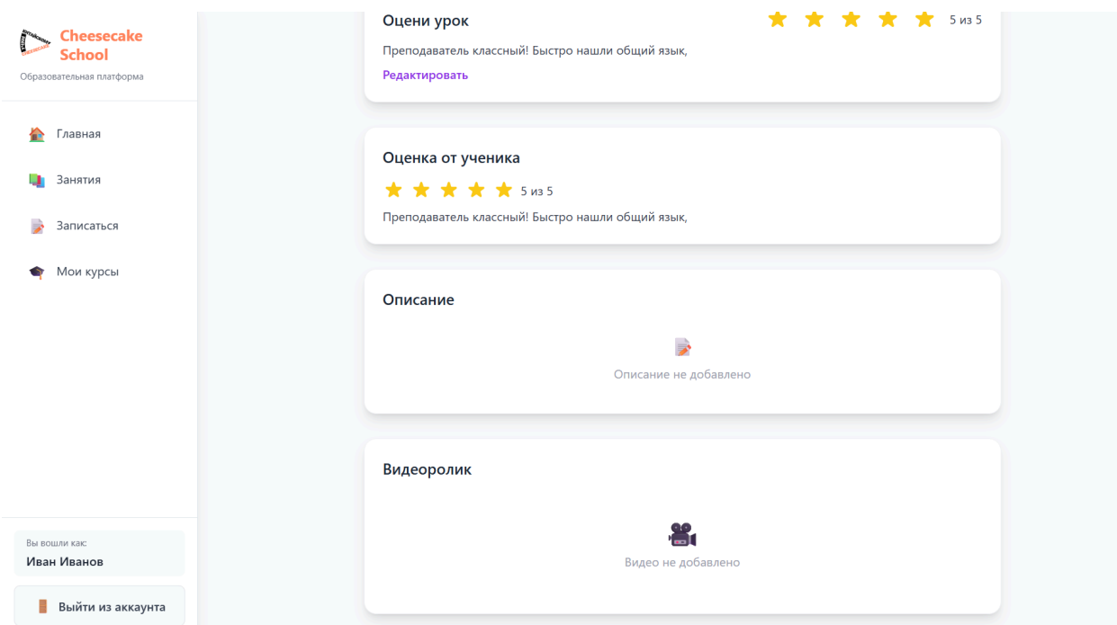
Рисунок 8 – Раздел Занятие
