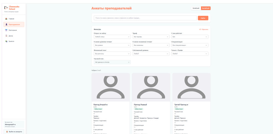
Рисунок 3 – Раздел Преподаватели
