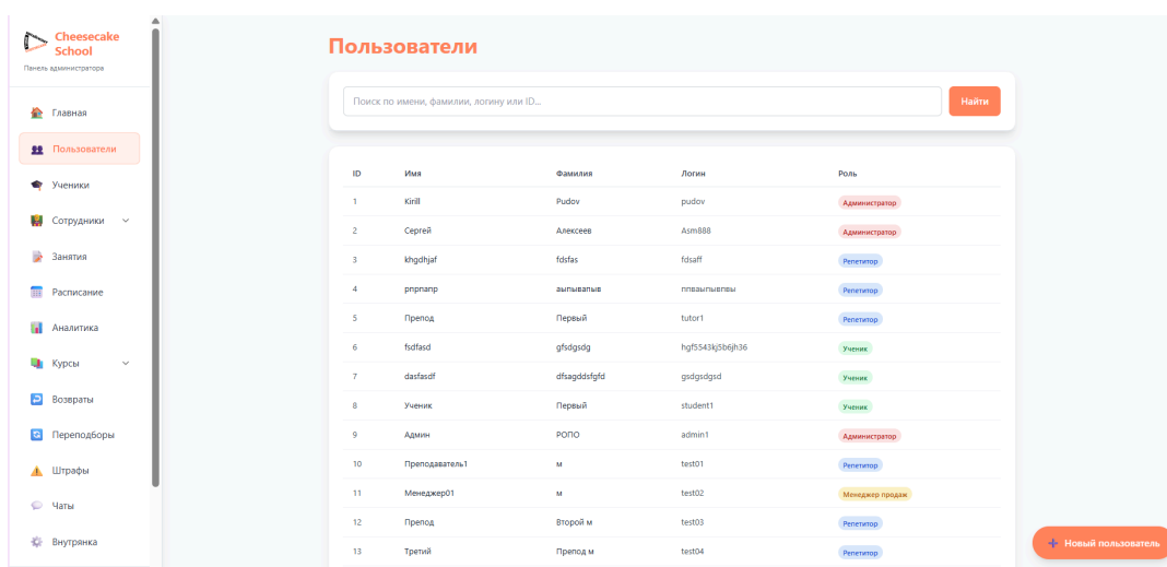
Рисунок 3 - Раздел Пользователи
