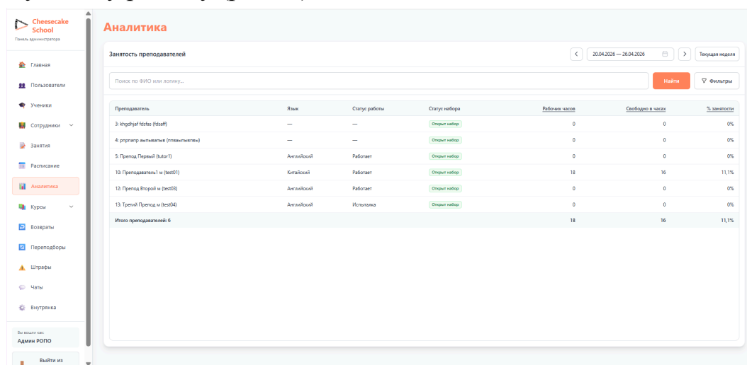
Рисунок 16 - Раздел Аналитика
