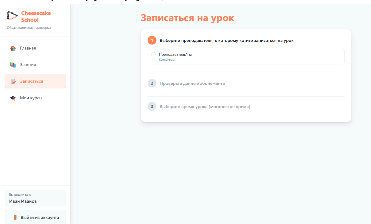
Рисунок 9 – Раздел Записаться
