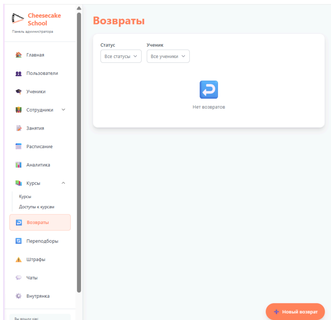
Рисунок 17 - Раздел Возвраты
