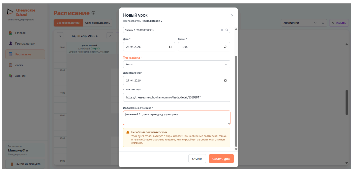
Рисунок 8 - Создание урока
