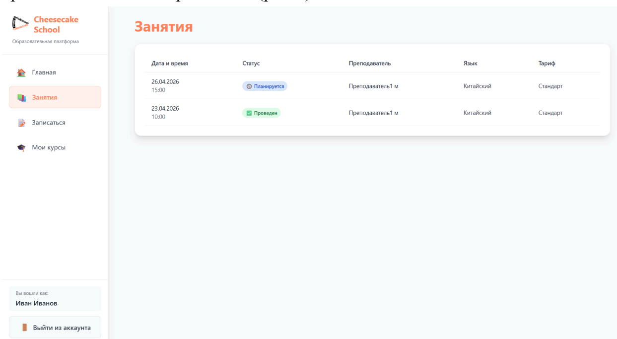
Рисунок 6 – Раздел Занятия
