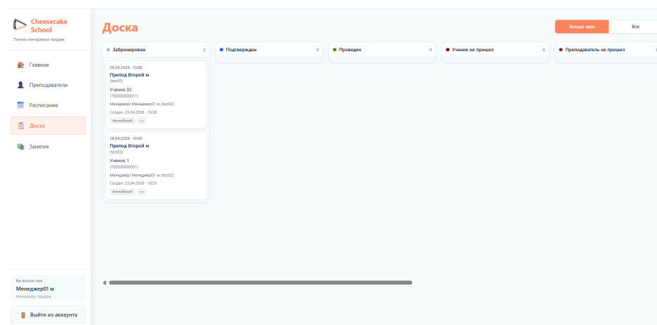
Рисунок 10 - Раздел Доска
