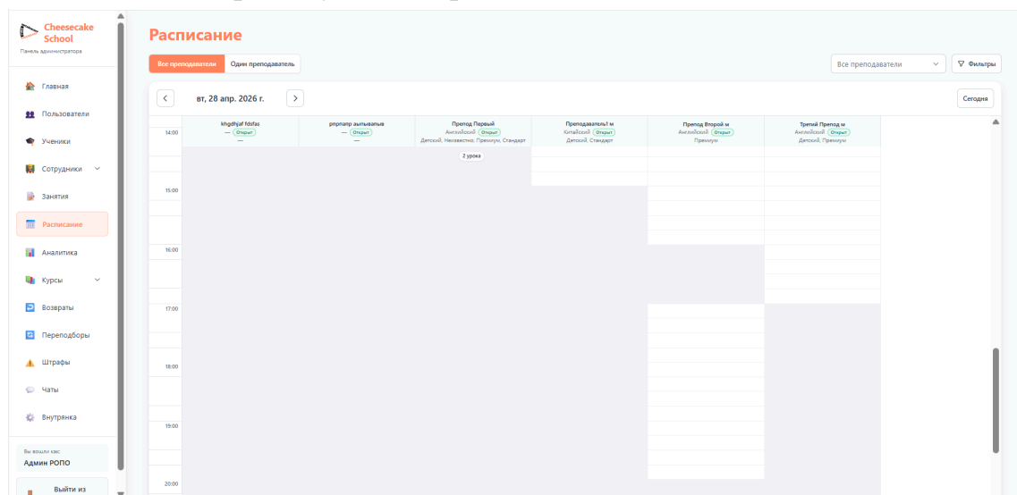
Рисунок 14 - Раздел Расписание
