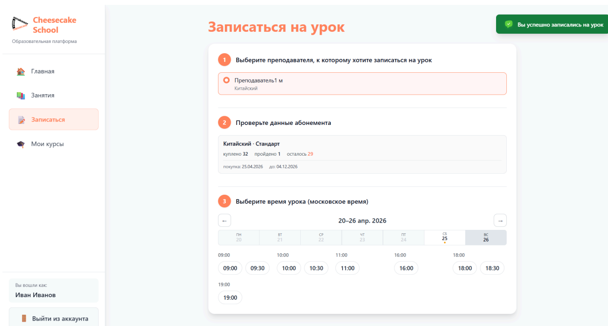
Рисунок 11 – Подтверждение записи
