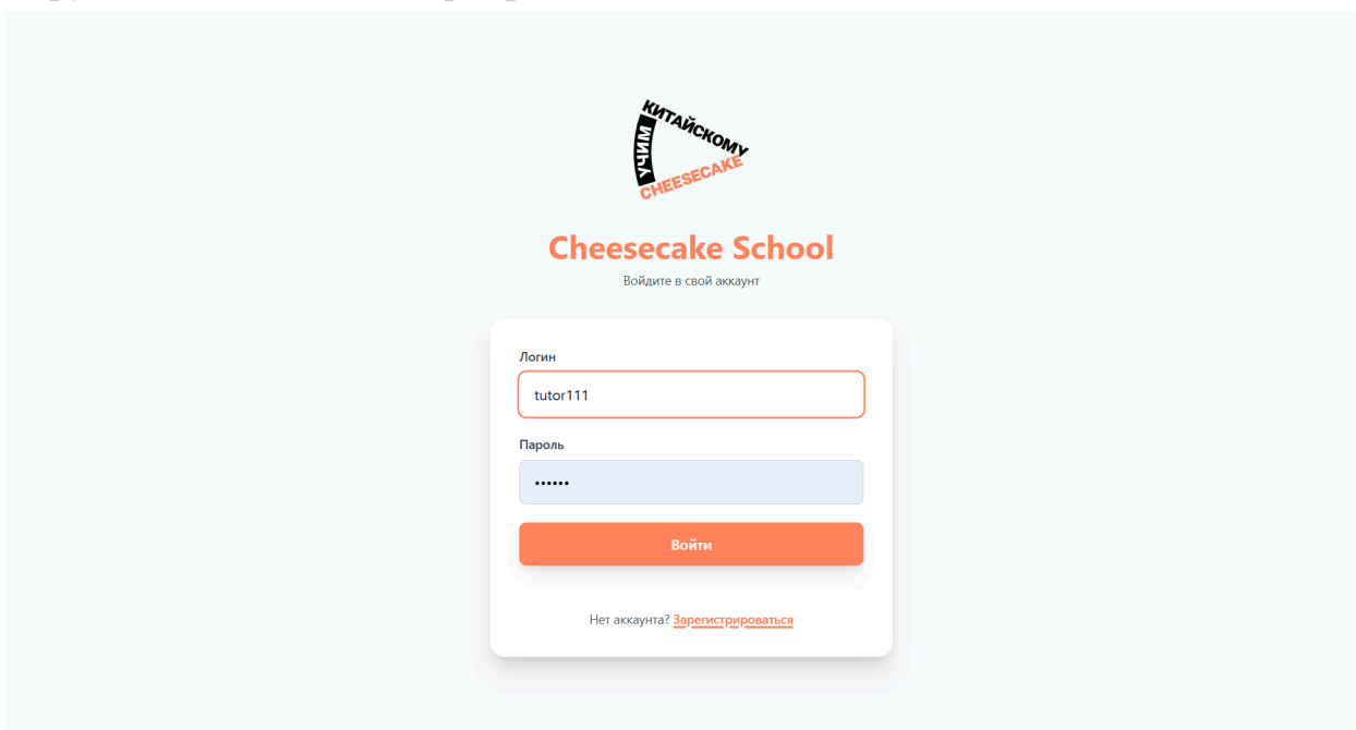
Рисунок 1 – Страница авторизации
