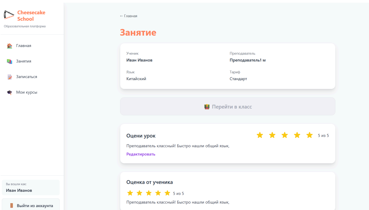
Рисунок 7 – Раздел Занятие
